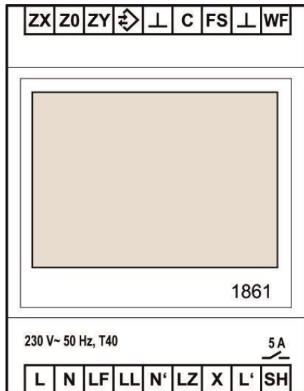
Klemmenbelegung 1861-ZSG
