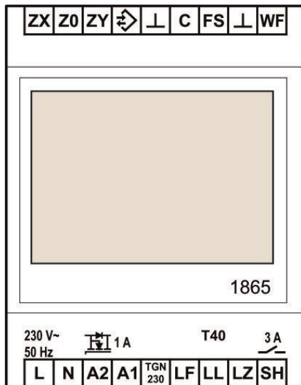
Klemmenbelegung 1865-ZSG
